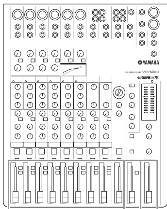
регуляторы уровня сигнала каналов
