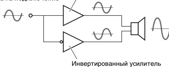
Инвертированный усилитель
